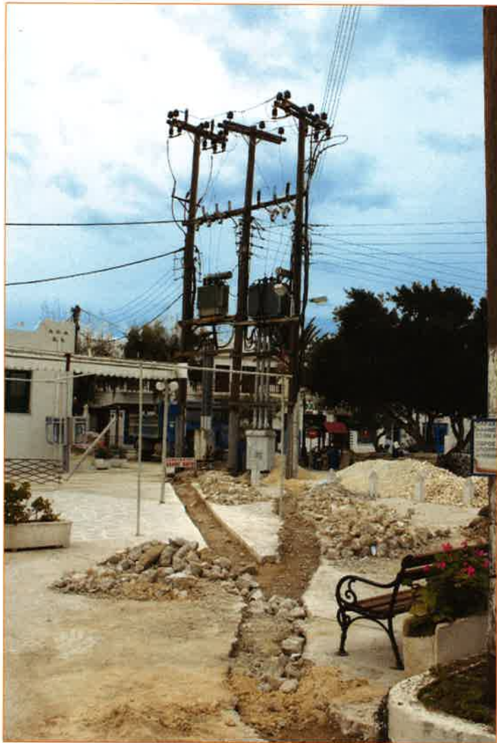
Αυτοί οι ανοιχτού τύπου και αντινοβολίας μετασχηματιστές κάποτε δέσποζαν στην πλατεία της Μαντώς
