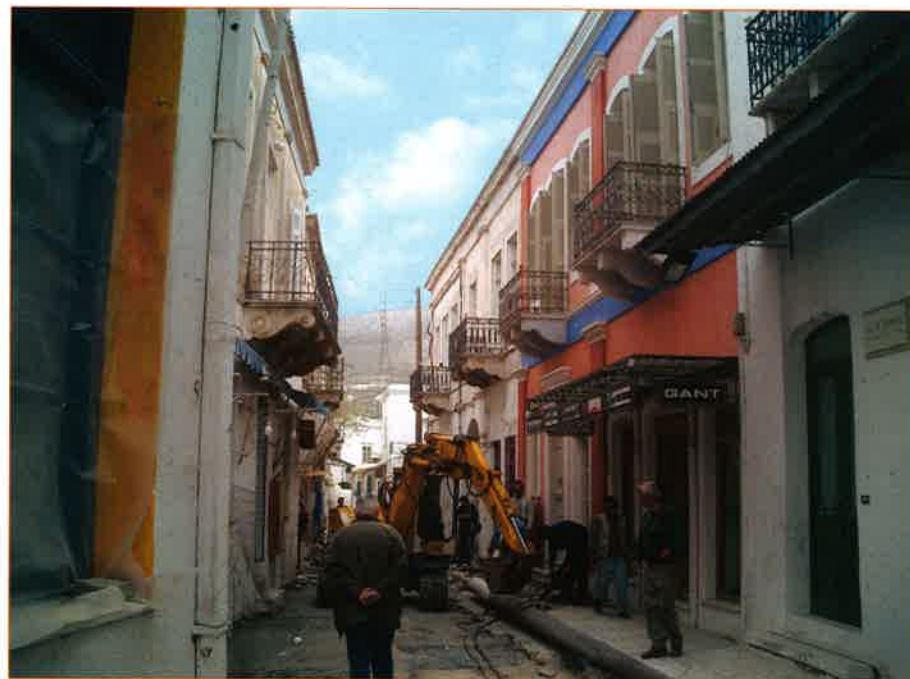
Υπογείωση δικτύων της ΔΕΗ στον παραδοσιακό οικισμό της Παροιτιάς
